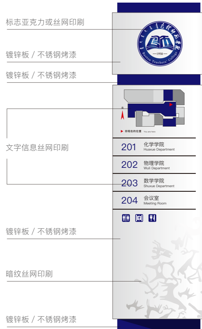
正视图
